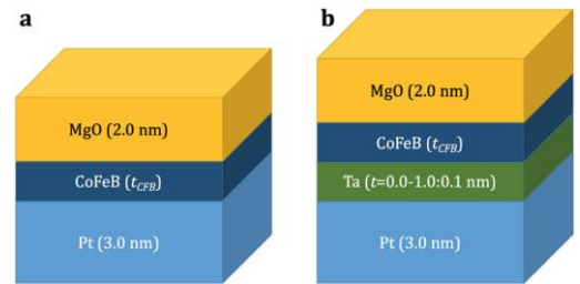
Şekil 1: Katmanlı film yapılarının şematik gösterimi a) Ta katmanı olmadan, b) farklı kalınlıklarda Ta katmanlı yapı
