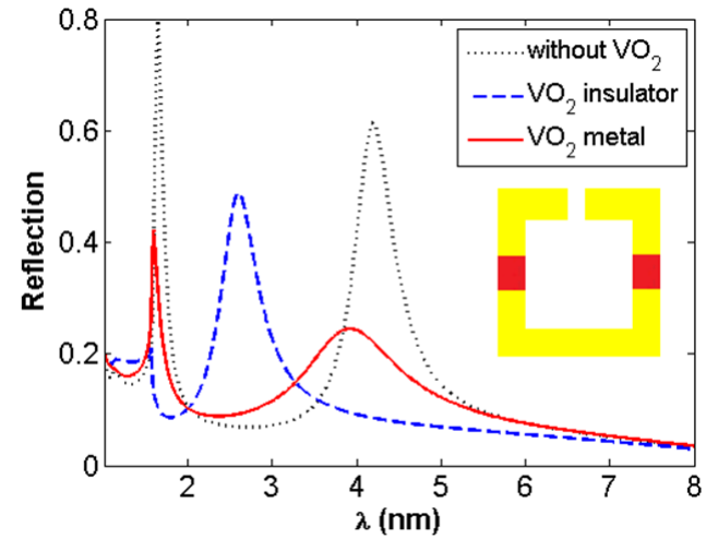
Şekil 1: VO 2 'nin bulunmadığı altın SRR dizisi (noktalı-siyah) ve VO 2 'nin varlığı (kesikli mavi yalıtkan fazı ve katı-kırmızı metal fazı) için yansımaları görülmektedir. İç metinde, dikkate alınan yapıların birim hücre şematik olarak gösterir. Boşluğun genişliği ve SRR'nin kolları 100 nm, kolların uzunluğu 460 nm, birim hücre boyutu 900x900 nm 2 ve altının kalınlığı 70 nm'dir. Düzlem dalgası olayı simülasyondaki SRR kollarına dik elektrik alanı dizisidir.
