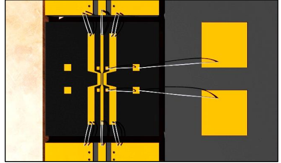
Şekil 1: Spin pompalama cihazının bir tasarımı.
