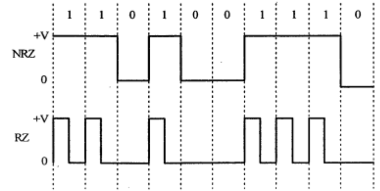
Şekil 4.2. Tek-kutuplu işaretleşme.
