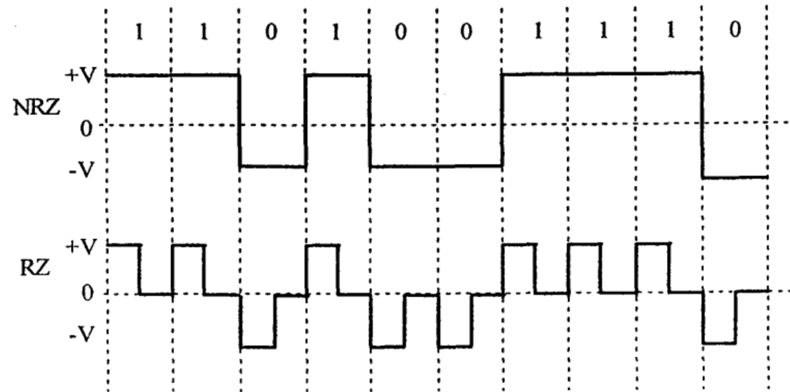
Şekil 4.6. Kutuplu işaretleşme NRZ ve RZ dalga biçimleri.
