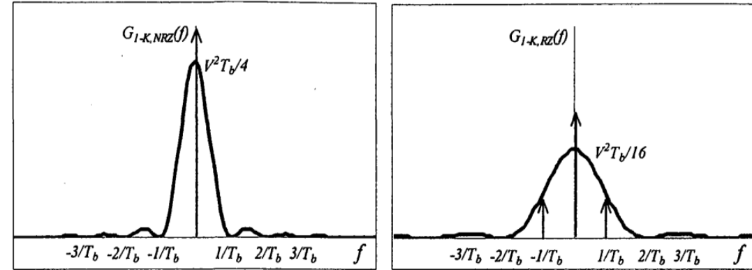
Şekil 4.3. Tek-kutuplu NRZ ve RZ işaretleşmesi için güç spektral yoğunlukları.
