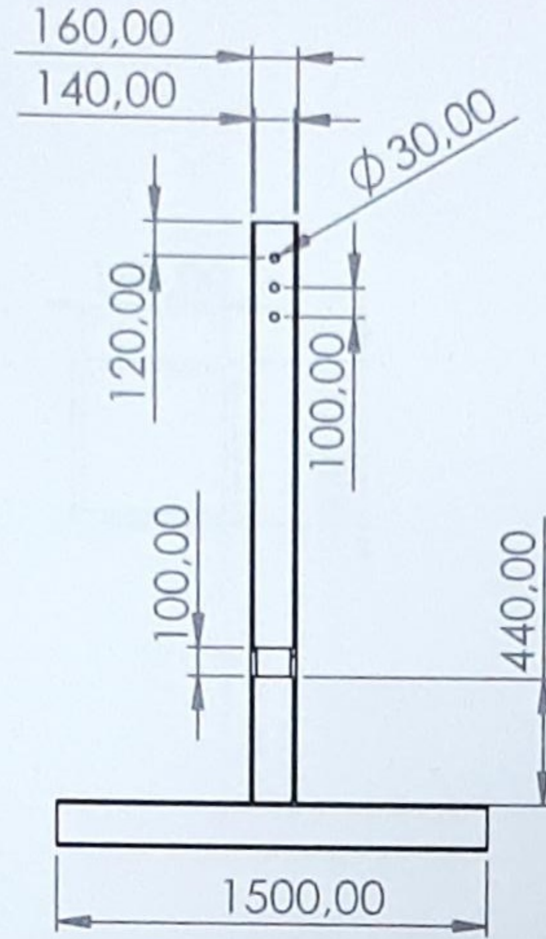
KESIT B-B ÖLÇEK 1 : 35
